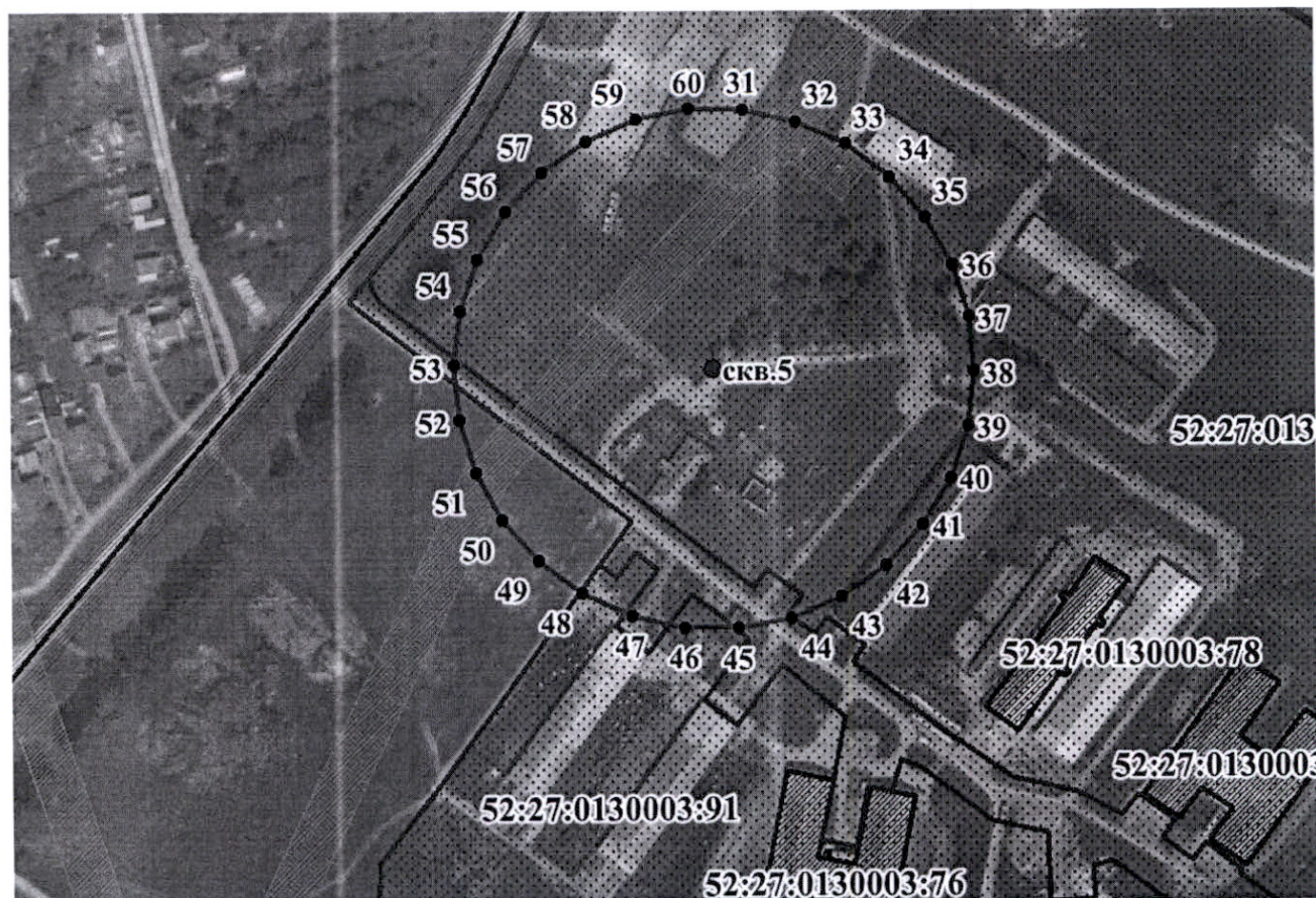
Координаты характерных точек границы третьего пояса ЗСО скважины № 5 ООО «Бармино» Лысковского муниципального района Нижегородской области
