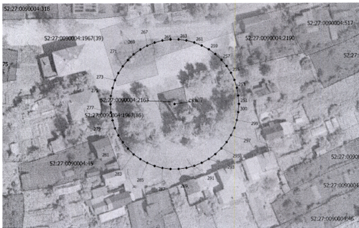
Координаты характерных точек границы второго пояса ЗСО водозаборной скважины № 7 МУП «Лысковокоммунсервис» в г. Лысково Нижегородской области
