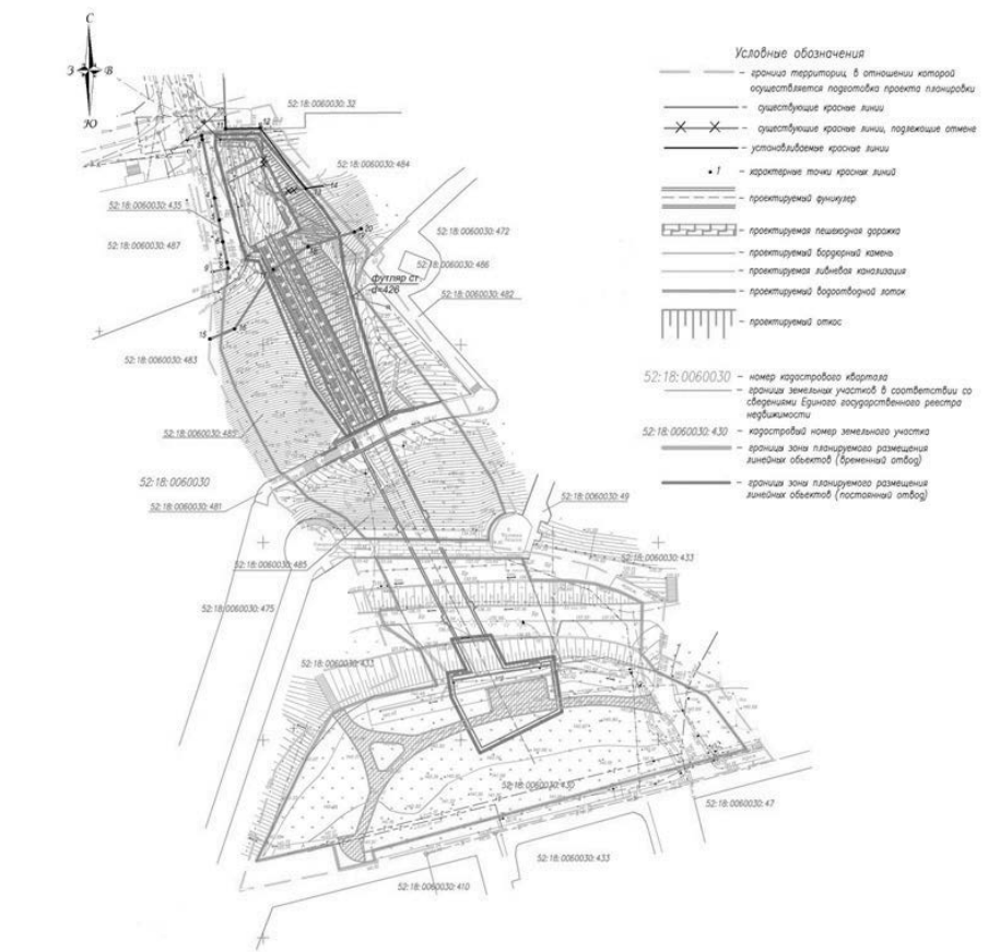
II. Чертеж границ зон планируемого размещения линейного объекта
