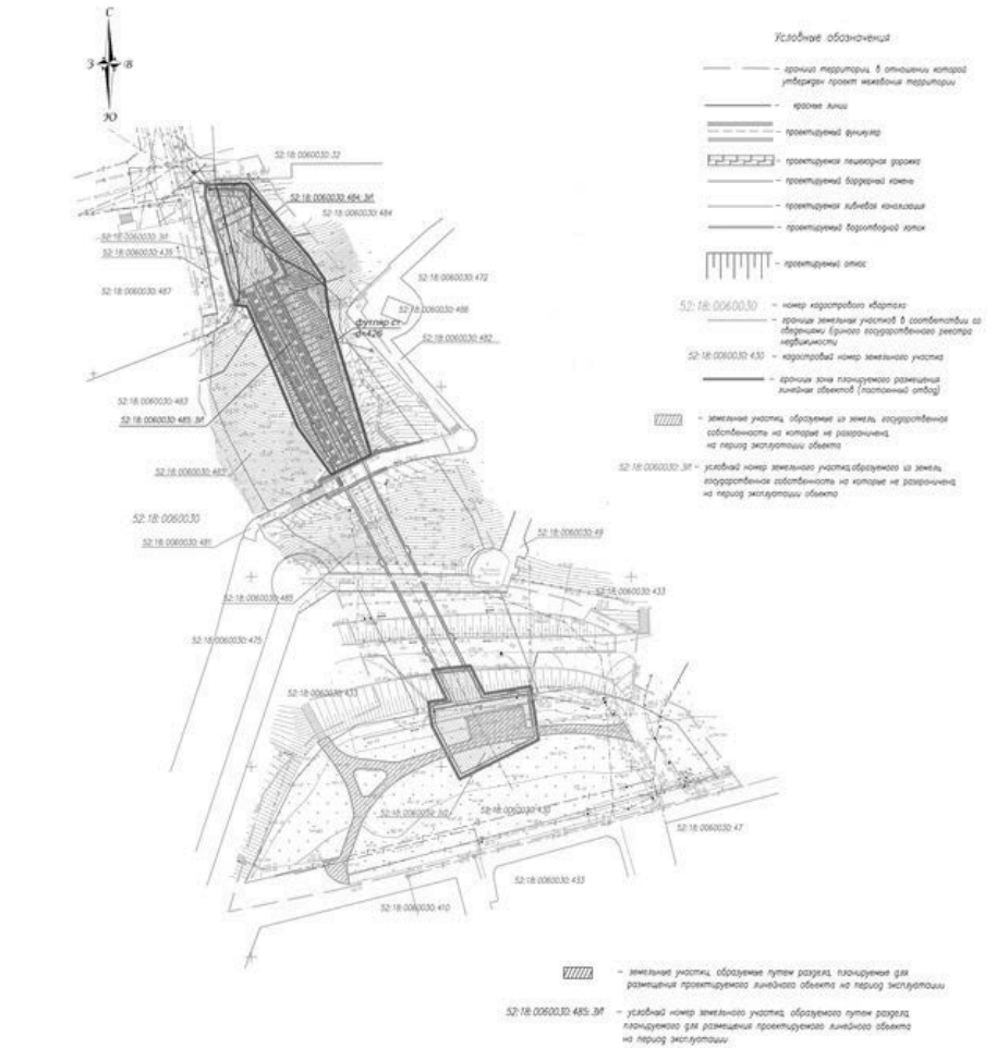
V. Чертеж межевания территории на период эксплуатации объекта
