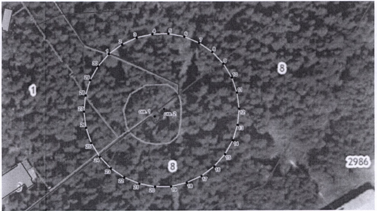
Координаты характерных точек границы первого пояса ЗСО скважин № 1 и № 2
