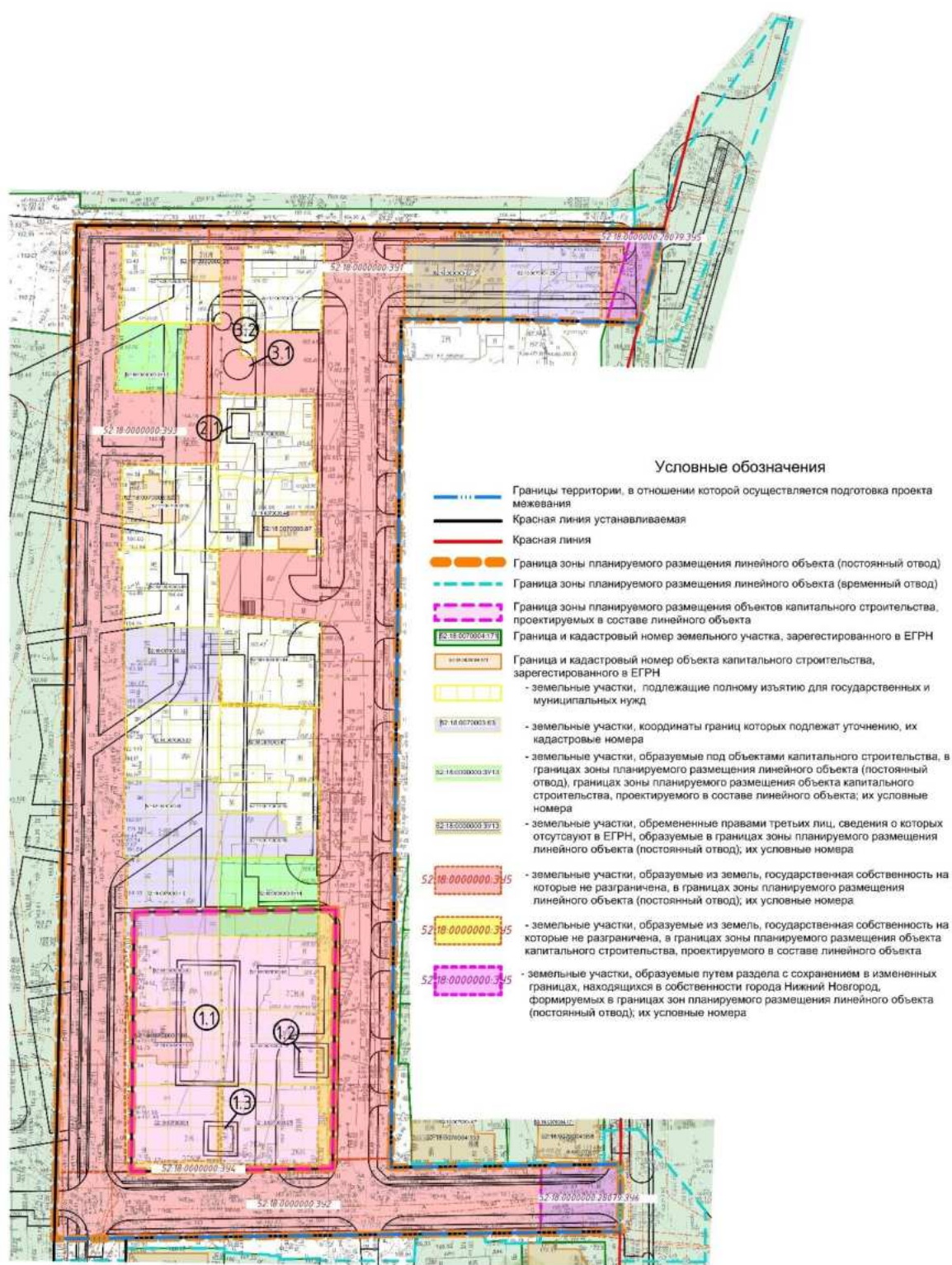
Экспликация проектируемых зданий и сооружений
