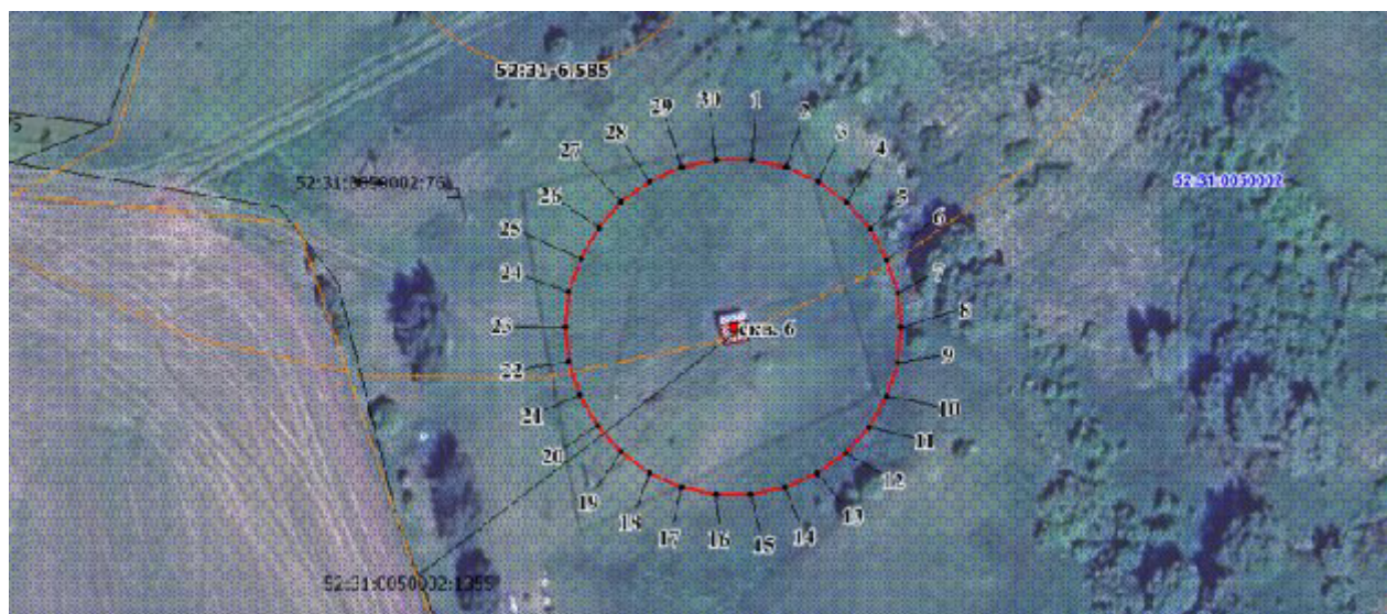
Координаты характерных точек границы первого пояса ЗСО скважины № 6
